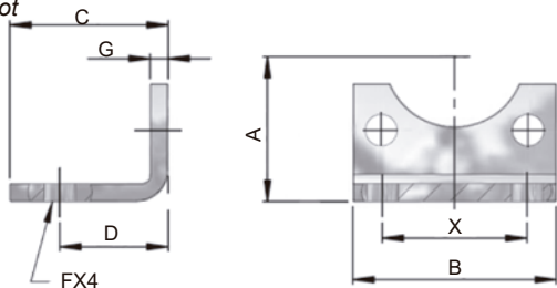
Pata fijación Axial foot
