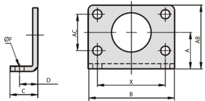
Placa fijación Axial foot
