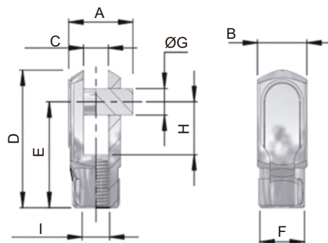
Horquilla Rod clevis
