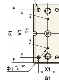
4-J Agujero pasante
